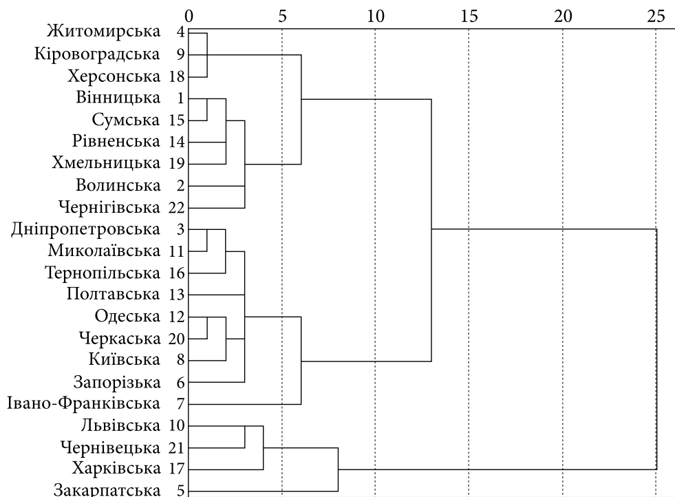
Рис. 5. Дендрограма кластеризації регіонів України методом внутрішньо групових зв'язків за показниками інтегрального ІРЛР за 2004—2017 рр.
